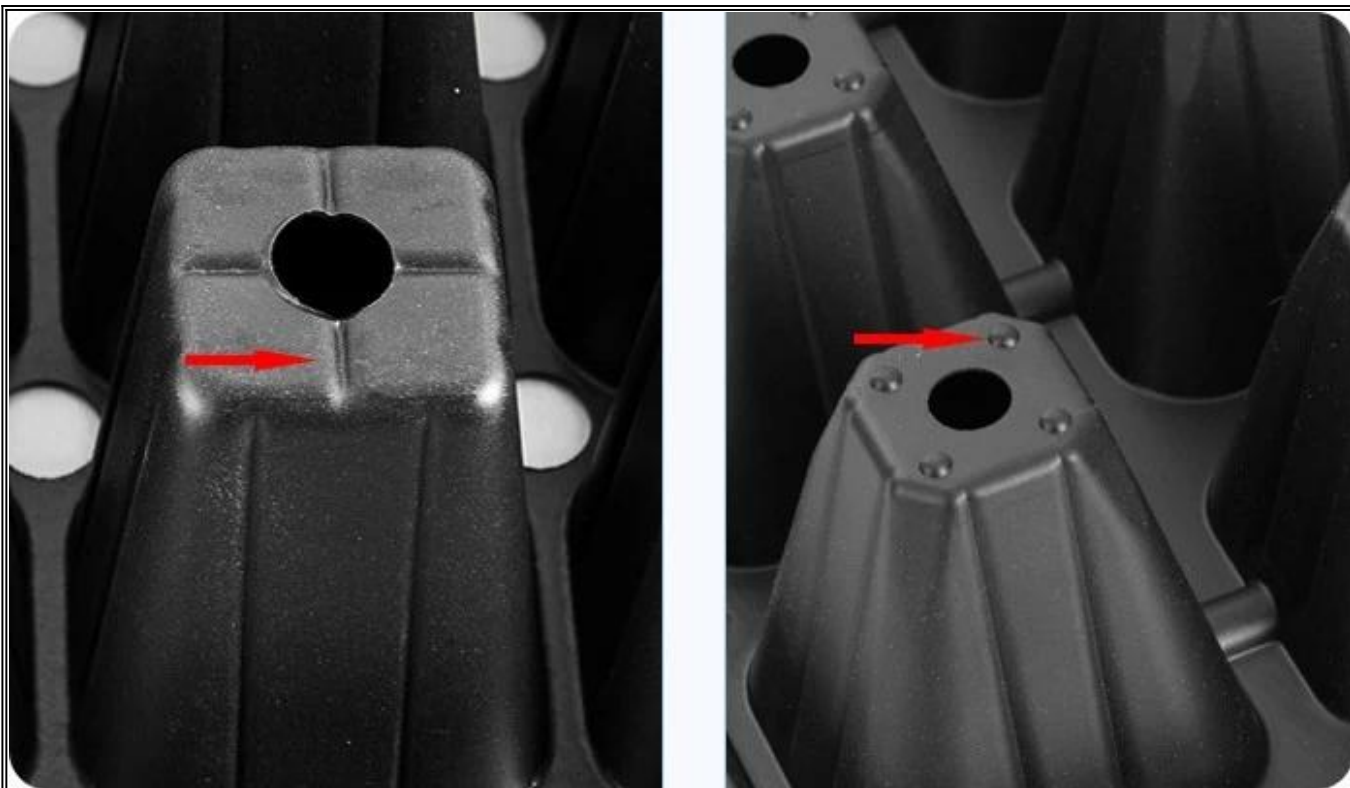
Нижний дизайн ячейки - Дизайн небольших канавок или выпуклостей на дне может привести к быстрому просачиванию воды из лотка для ячеек.
