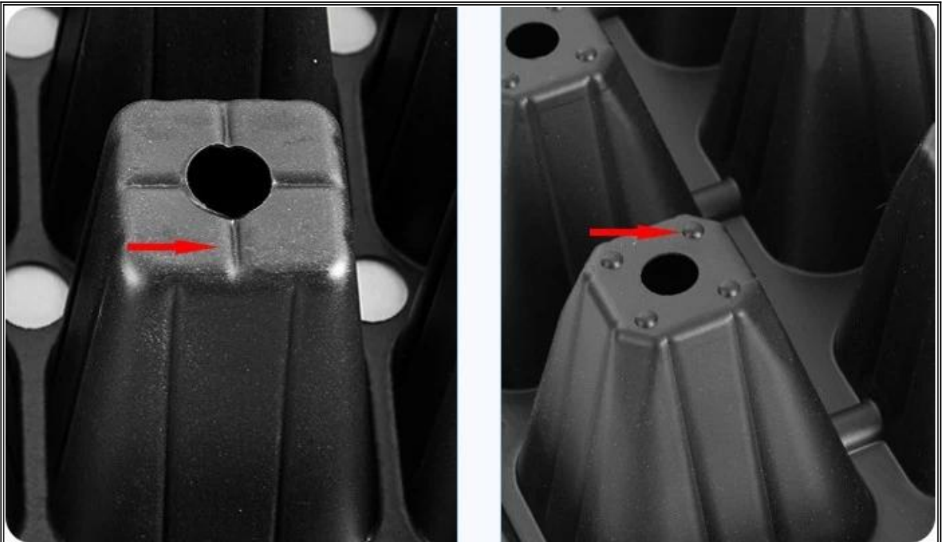
圖 2 顯示了模具的缺陷，紅箭頭指向缺陷位置。
